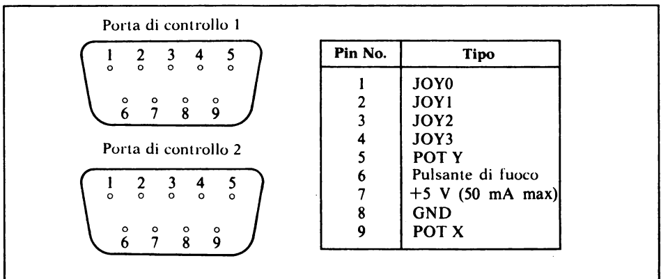
Figura C.1. Pin della porta per i joystick
