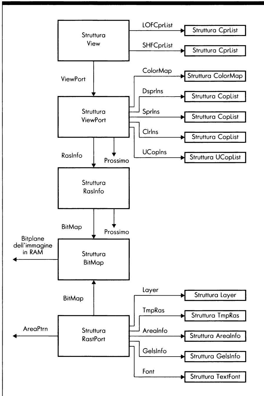
Figura 2.2: Legami fra le principali strutture previste dalla libreria Graphics
