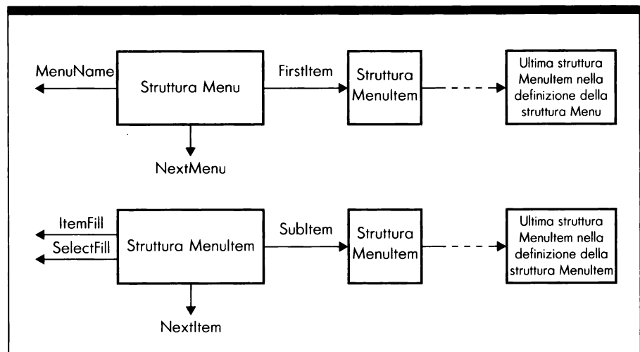
Figura 6.6: Collegamenti fra strutture per le strutture Menu e MenuItem
