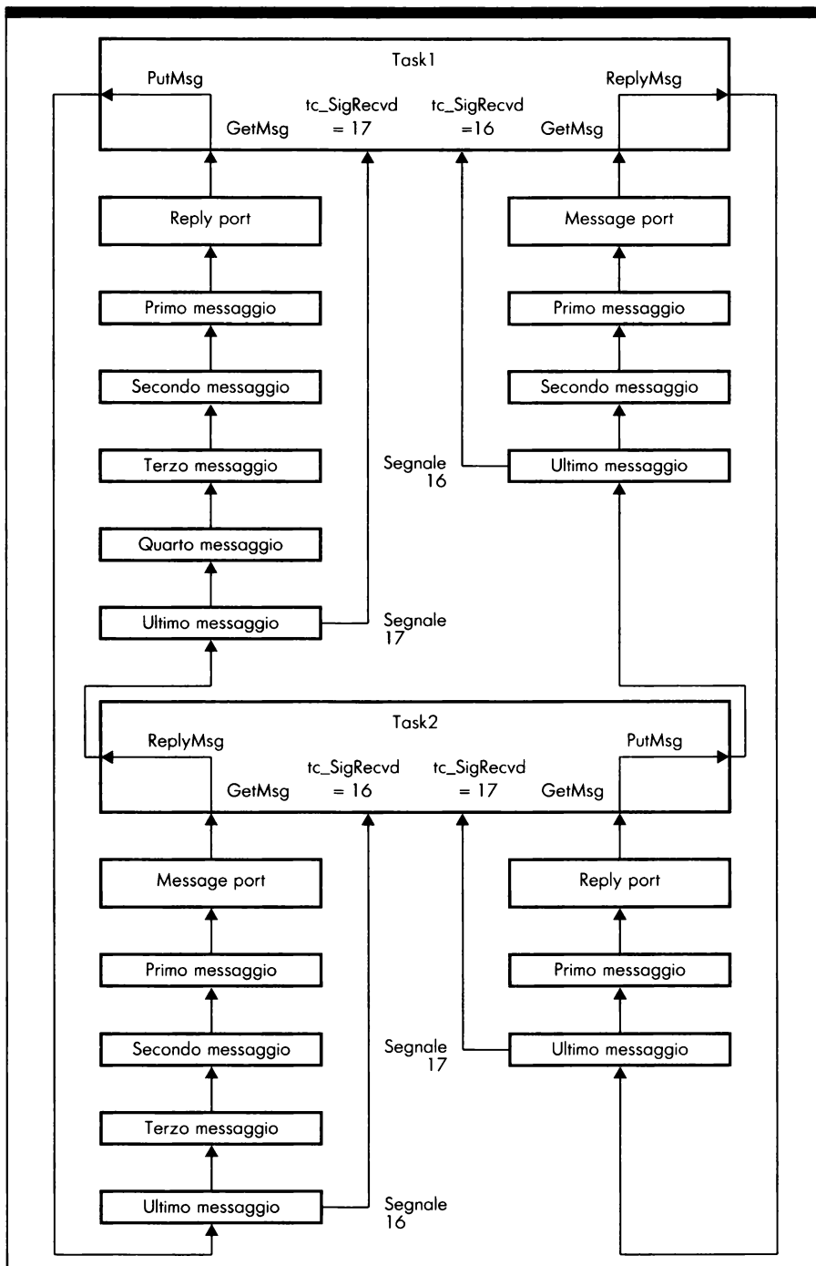
Figura 1.1: Task, message port, messaggi e segnali
