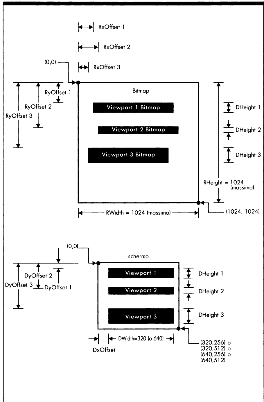
Figura 2.4: Bitmap, viewport, offset nella view e dimensioni
