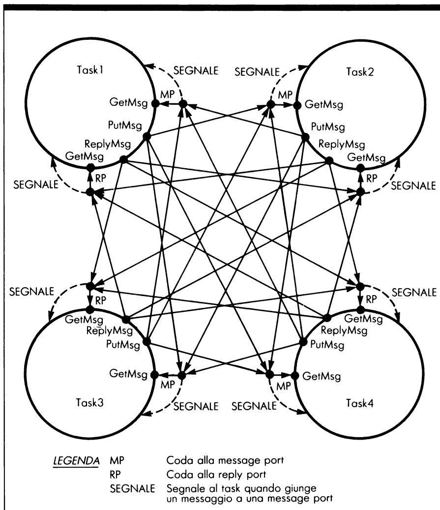
Figura 1.2: Diversi task, message port, messaggi, e segnali
