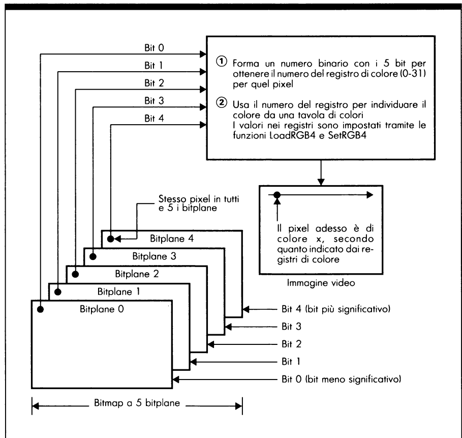
Figura 2.1: Bitplane, bitmap, registri di colore e colori dei pixel
