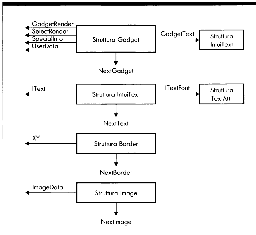
Figura 6.7: Collegamenti delle strutture Gadget, IntuiText, Border e Image
