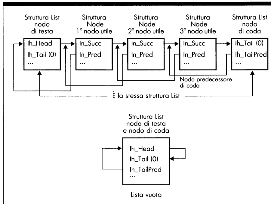
Figura 1.3: Organizzazione di una lista doppia con tre nodi (in alto) e vuota (in basso)
