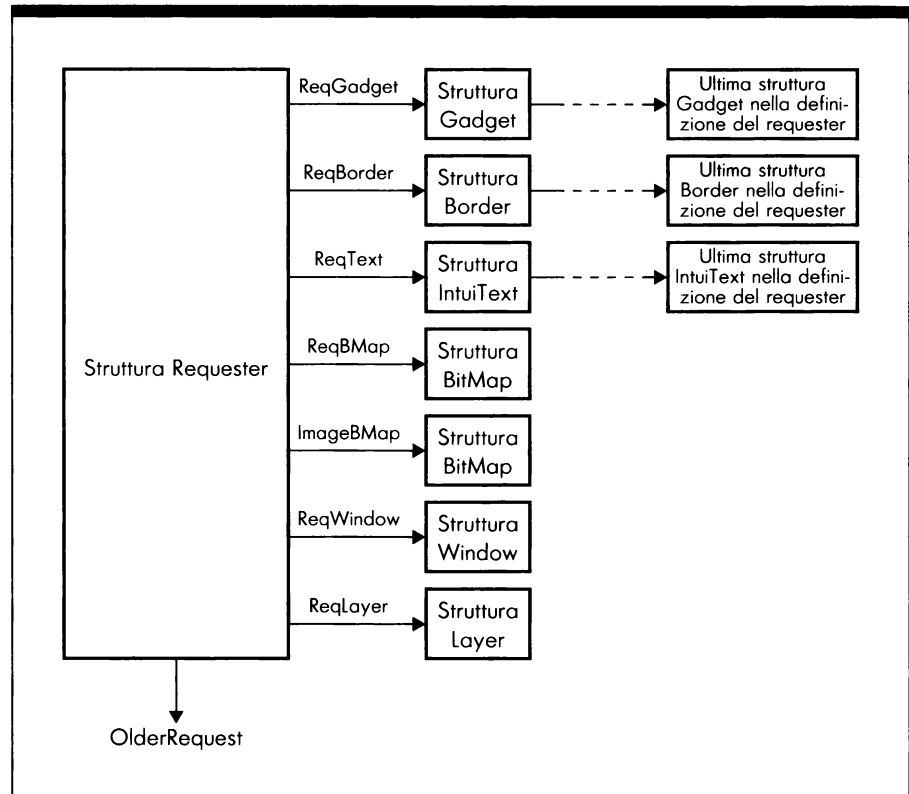
Figura 6.5: Collegamenti fra strutture per la struttura Requester
