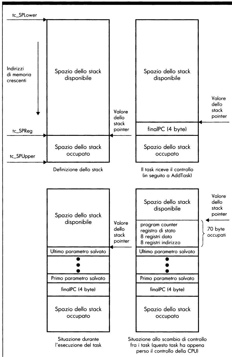
Figura 1.5: Comportamento dello stack del task
