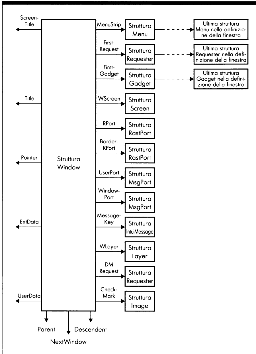
Figura 6.4: Collegamenti fra strutture per la struttura Window
