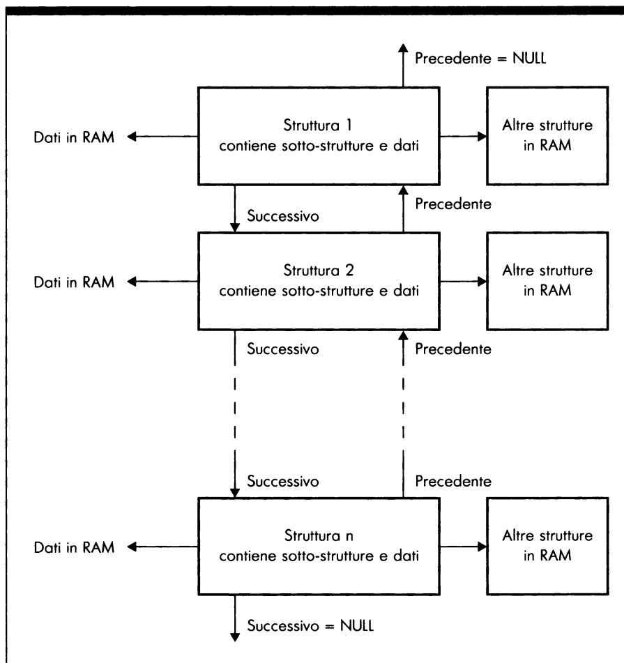
Figura I.1: Lista a doppia concatenazione
